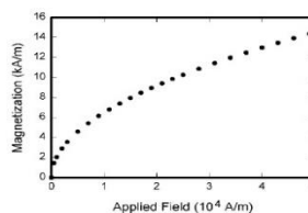
ภาพที่ 1 แสดงความสัมพันธ์ระหว่าง Applied Field กับ Magnetization ของวัสดุชนิด XYZ
